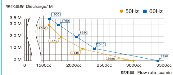
CH-525 Discharge Diagram 排水量
